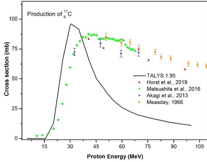
Figür 3. ^{11}\text{C} radyoizotop üretimi için ^{12}\text{C}(\text{p},\text{x})^{11}\text{C} reaksiyon tesir kesiti
